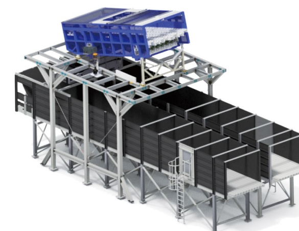
(定量供給機とバリスティックセパレーターとの組み合わせ)
